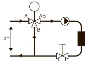
С. Схема с локальным циркуляционным насосом
