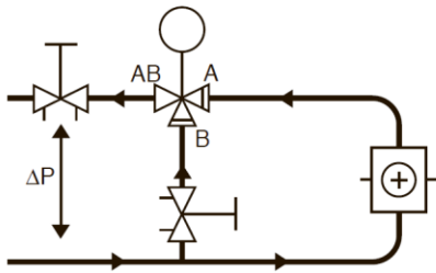
А. Схема без локального циркуляционного насоса
